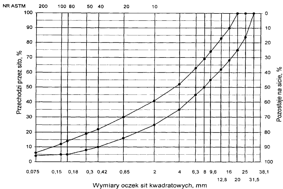
Rys. 11. Krzywe graniczne uziarnienia mieszanki mineralnej BA od 0 do 25mm do warstwy wiążącej, wyrównawczej i wzmacniającej nawierzchni drogi o obciążeniu ruchem od KR2 do KR6
