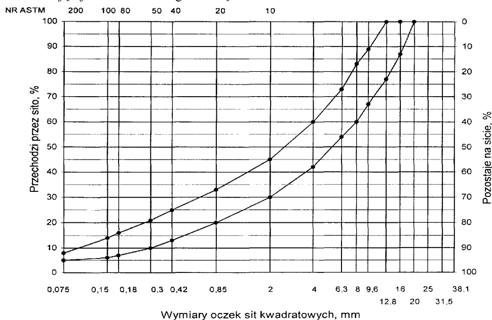
Rys. 12. Krzywe graniczne uziarnienia mieszanki mineralnej BA od 0 do 20mm do warstwy wiążącej, wyrównawczej i wzmacniającej nawierzchni drogi o obciążeniu ruchem od KR2 do KR6
