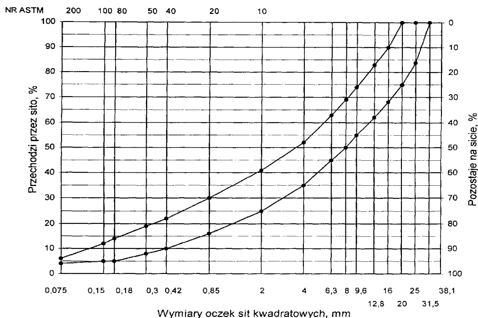
Rys. 12. Krzywe graniczne uziarnienia mieszanki mineralnej BA od 0 do 20mm do warstwy wiążącej, wyrównawczej i wzmacniającej nawierzchni drogi o obciążeniu ruchem od KR2 do KR6
