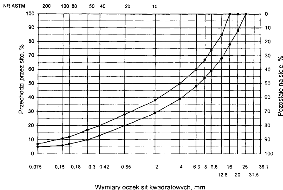
Rys. 4. Krzywe graniczne uziarnienia mieszanki mineralnej BA od 0 do 20mm do warstwy ścieralnej nawierzchni drogi o obciążeniu ruchem od KR2 do KR6
