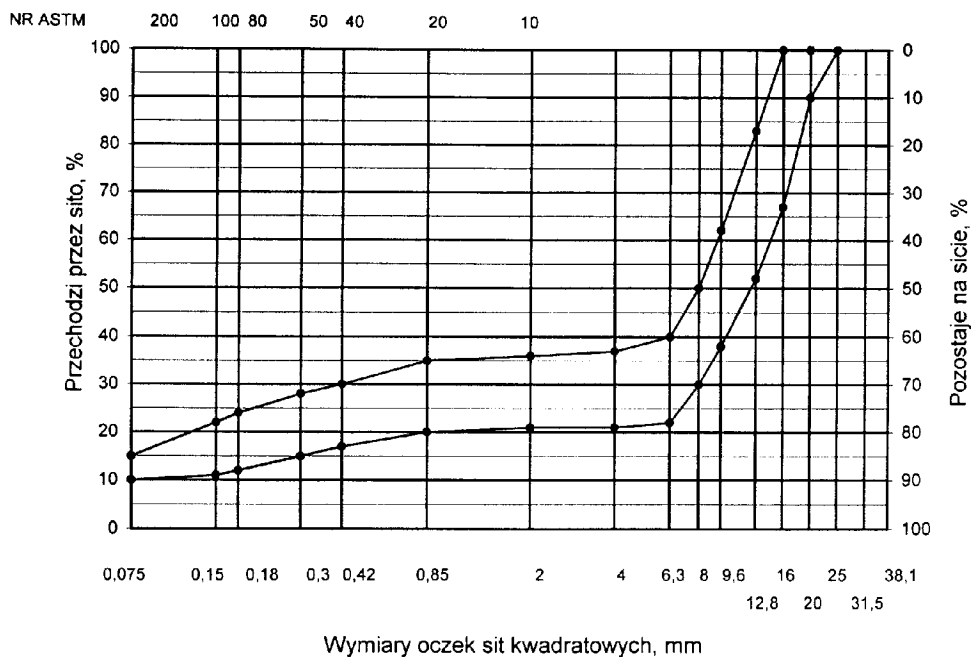
Rys. 5. Krzywe graniczne uziarnienia mieszanki mineralnej BA od 0 do 20mm (mieszanka o nieciągłym uziarnieniu) do warstwy ścieralnej nawierzchni drogi o obciążeniu ruchem od KR2 do KR6
